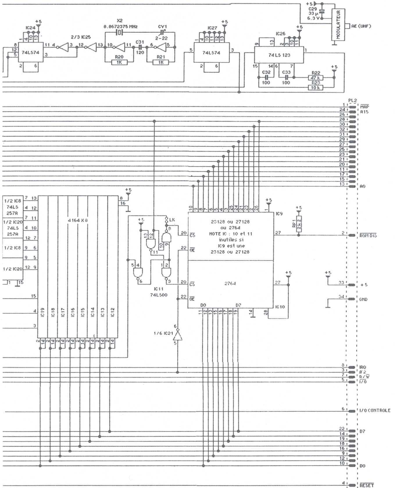
Schéma de l'ORIC 48 k
